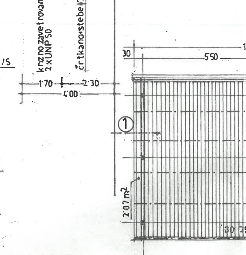
STREHA NAD VSTOPNO TOČKO TLORIS SPUŠČENEGA STROPA
