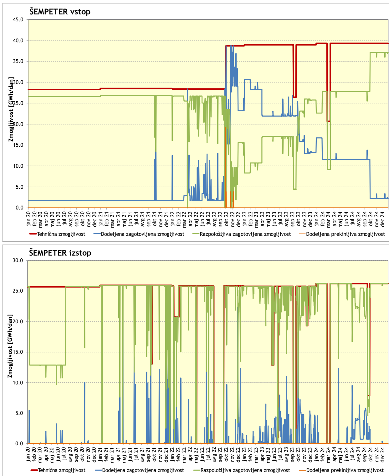
Slika 26. Prenosne zmogljivosti in stanje na mejni povezovalni točki Šempeter v letih 2020-2024
